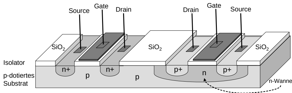
Abb. 5.1: n-MOS-Transistor und p-MOS Transistor auf gemeinsamem p-Substrat
