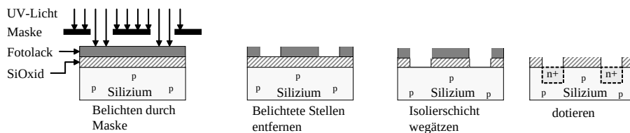
Abb. 5.3: Photolithographische Chipbearbeitung
